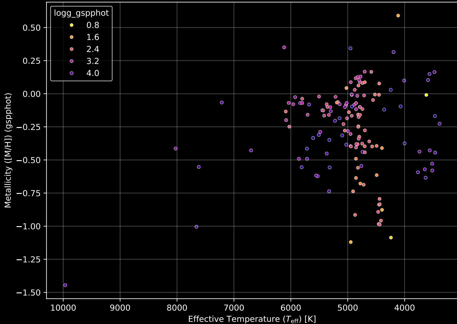
APOGEE DR17 Field: [K2_C2_350+23] Stellar Population Parameters (n= 148)
